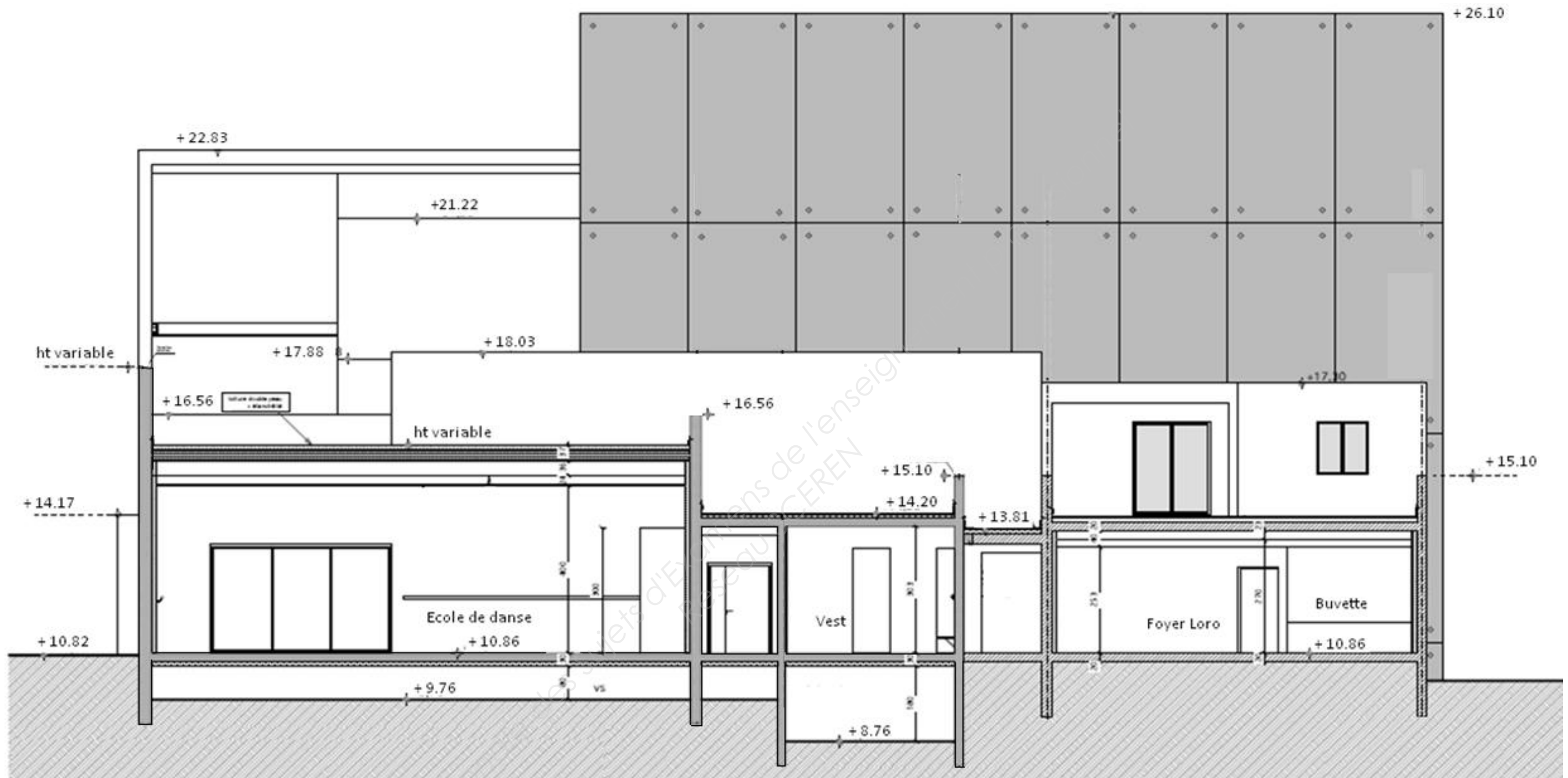
COUPE BB
